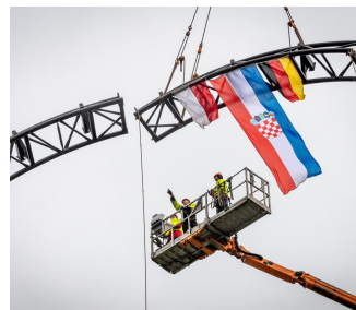
Die Schiene ist 6,71 Meter lang und wiegt 1,9 Tonnen – dabei repräsentieren die Flaggen den deutschen Hersteller MACK Rides, den neuen kroatischen Themenbereich und die polnische Aufbau-Crew von RCS.
